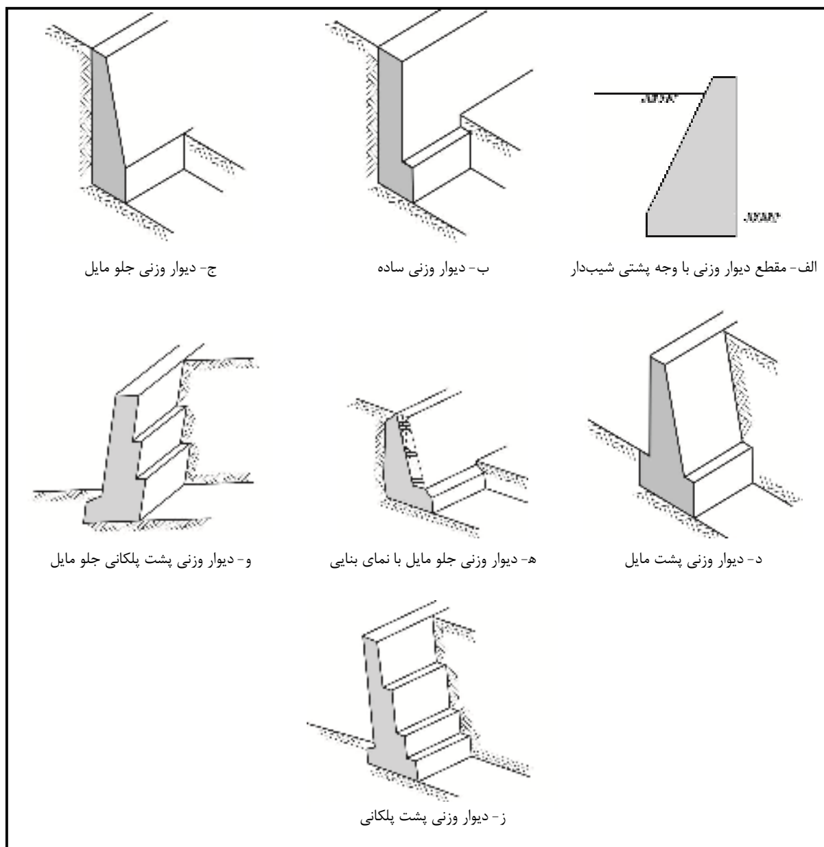
شکل ۱-۲- دیوارهای حایل صلب، دیوارهای حایل وزنی
