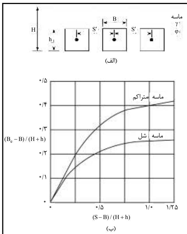
شکل ۱۰-۲۵- (الف) حالت واقعی نصب مهارها، (ب) تغییرات (B_e - B)/(H + h) در مقابل (S' - B)/(H + h) برپایه تحلیل اوسن و استرومن
