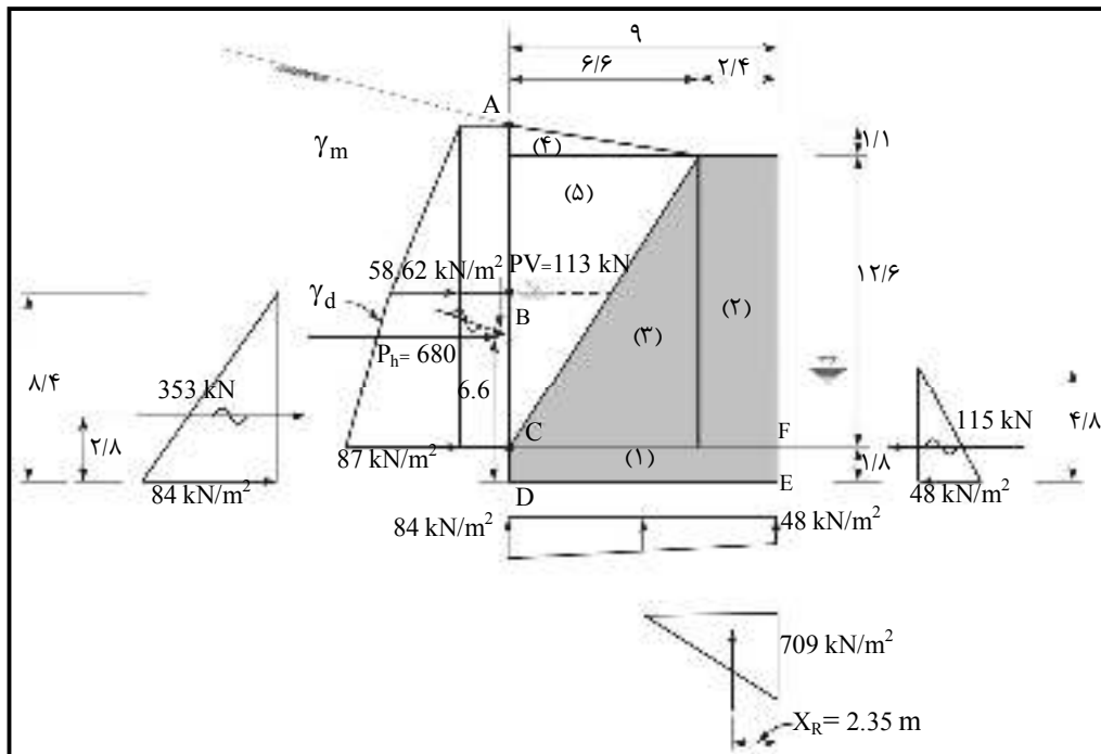
شکل ۸-۴- نمودار نیروها
