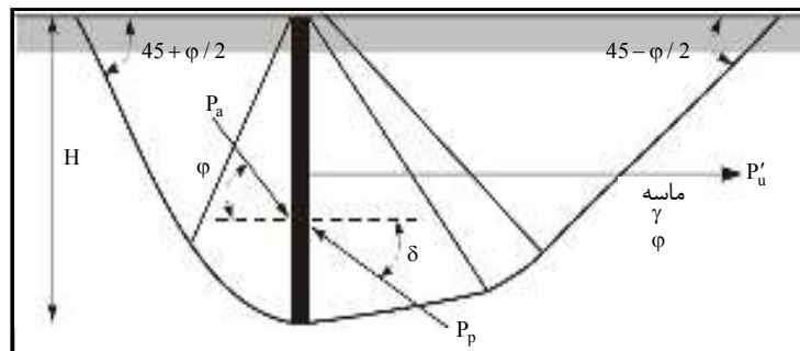
شکل ۱۰-۲۲- حالت پایه - صفحه‌ی مهاری پیوسته قائم در خاک دانه‌ای
