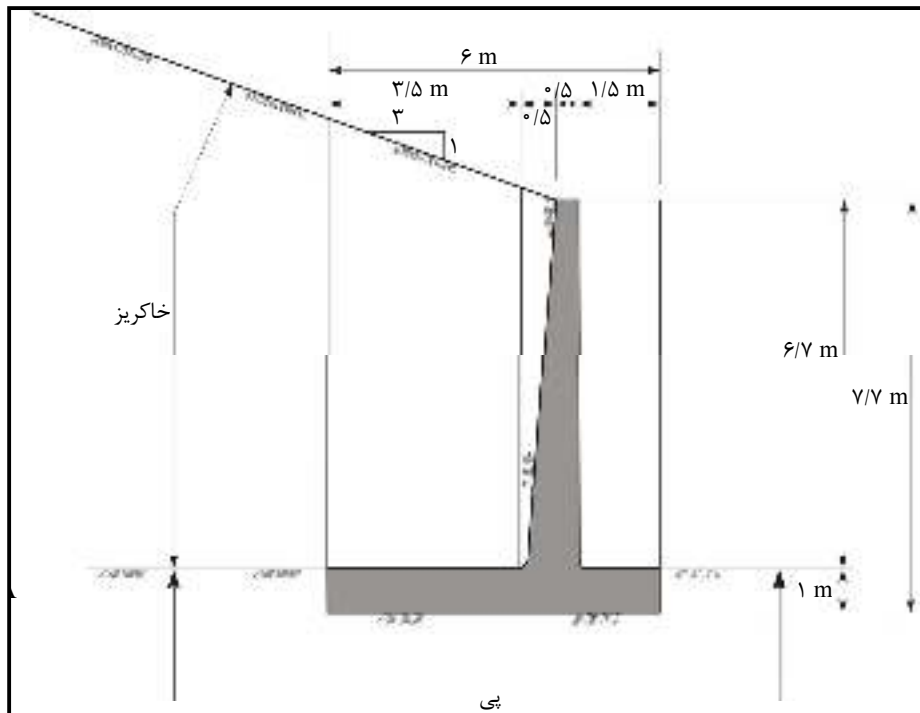
شکل ۹-۳- مقطع دیوار
