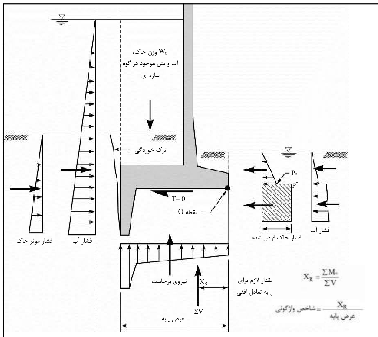
شکل ۴-۵- نیروهای وارده در تحلیل واژگونی دیوارها با پایه افقی و زبانه‌ی برشی
