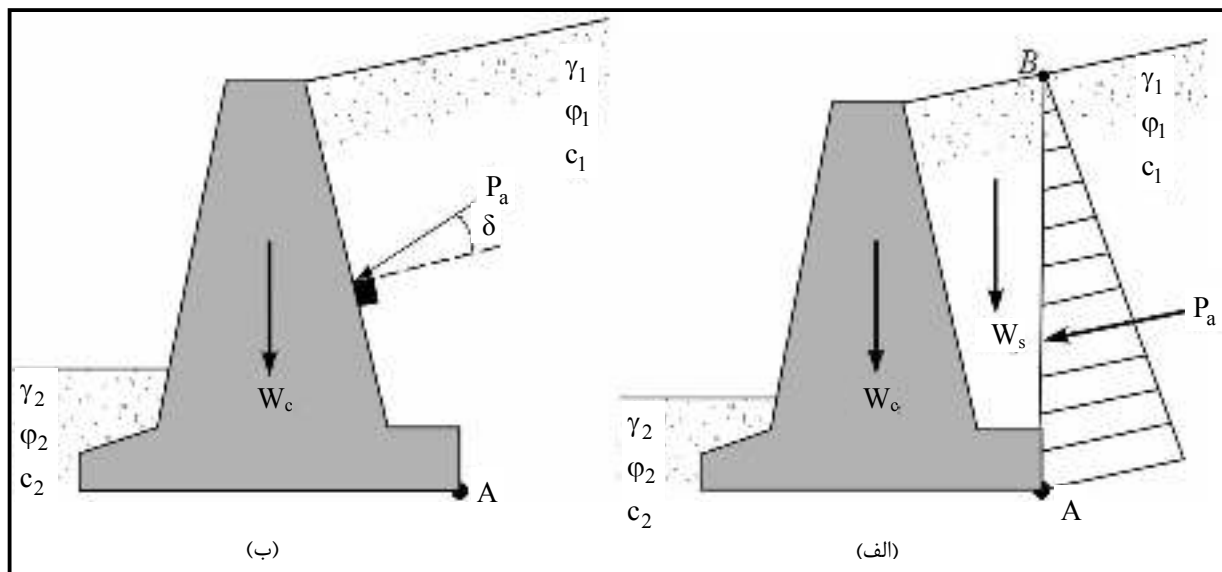
شکل ۳-۶- موقعیت اعمال برآیند فشار جانبی در نظریه رانکین (الف) و کولمب (ب)
