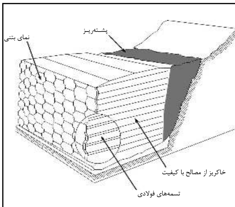
شکل ۱۲-۱- دیوار خاک مسلح
