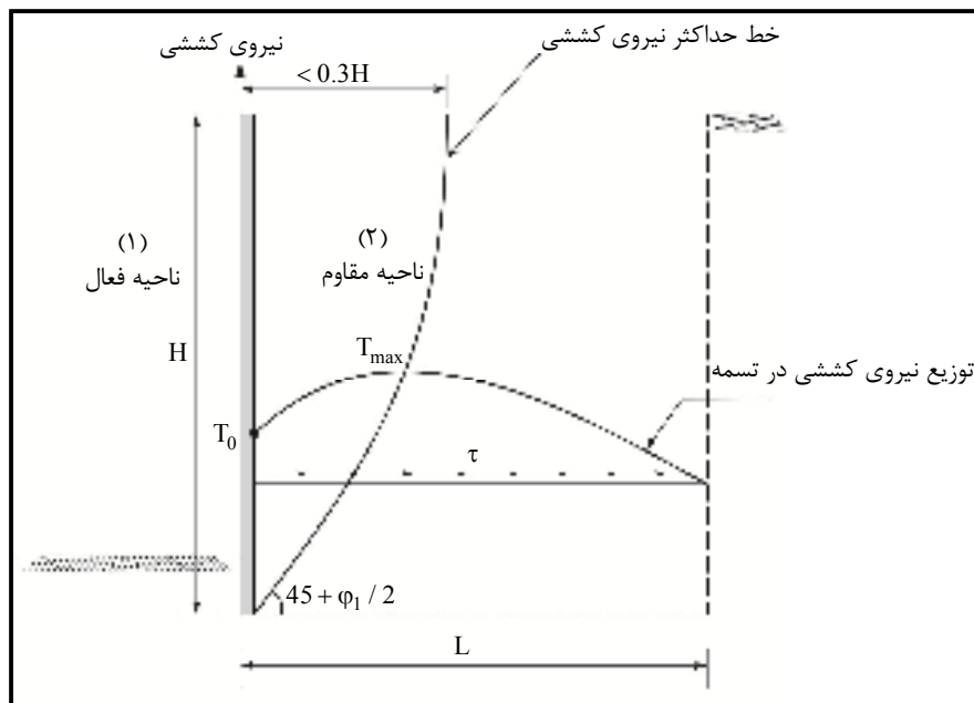
شکل ۱۰-۱۲- خط کشش حداکثر و نواحی فعال و مقاوم
