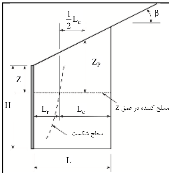
شکل ۱۳-۲۰- تنش قایم اسمی در تراز مسلح‌کننده در ناحیه مقاوم زیر خاکریز شیب‌دار
