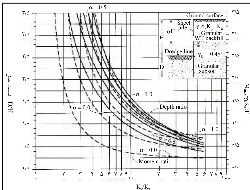
شکل ۱۰-۳۰ - سپر طره‌ای در بستر و خاکریز دانه‌ای، \gamma_b = 0.4\gamma
