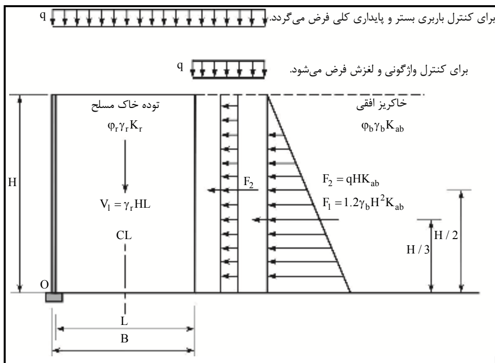
شکل ۱۳-۶- دیوار قایم و خاکریز افقی پشت دیوار
