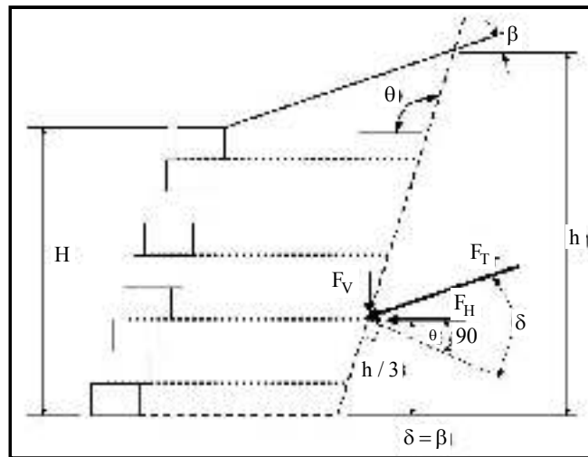
شکل ۱۳-۹- دیوار مایل (غیر قائم) با یا بدون خاکریز شیب‌دار
