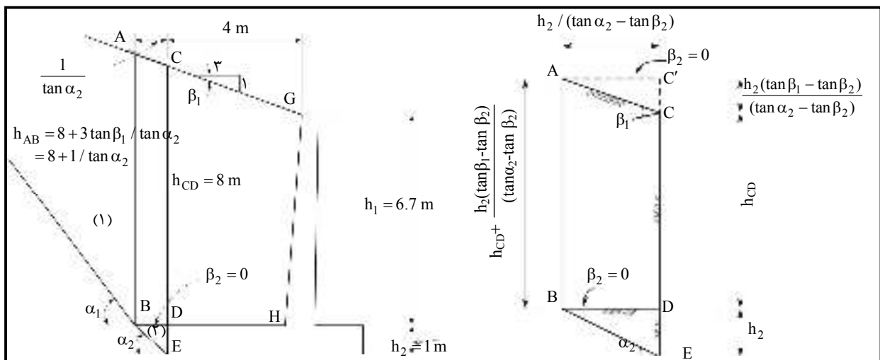
شکل ۹-۴- مشخصات گوه (۲)
