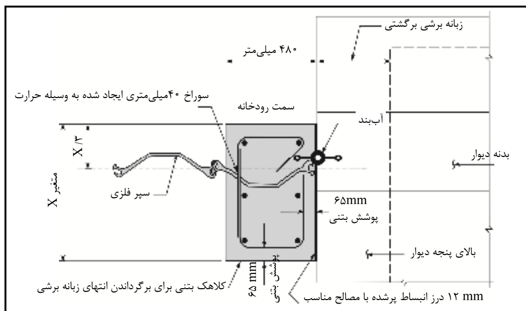
شکل ۷-۹- جزییات تیپ اتصال دیوار T با واحد اتصال (مقطع A-A شکل ۷-۸)
